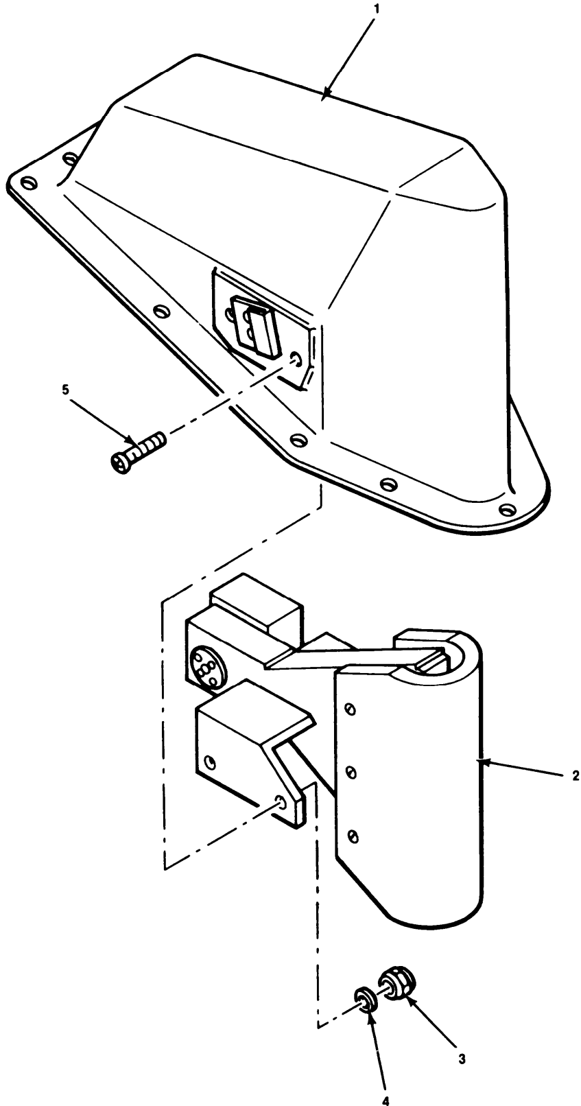
Figure 16. Antenna AS-3007 /ALQ-136 (V)
